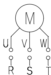
配線図 (L品)
