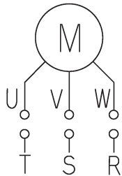
配線図 (L品)
