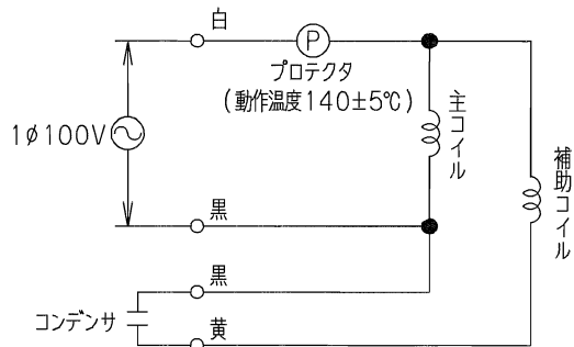
配線図
