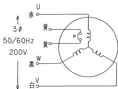
配線図
