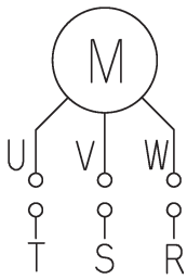
配線図
