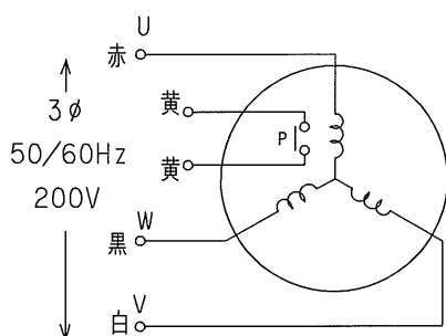
配線図
