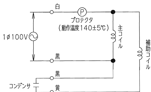
配線図
