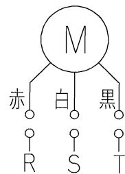
配線図
