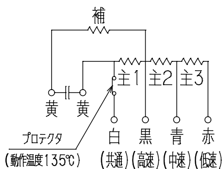
配線図
