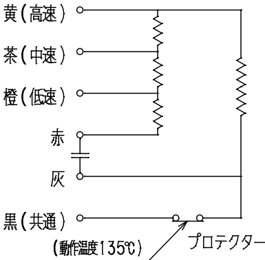
配線図
