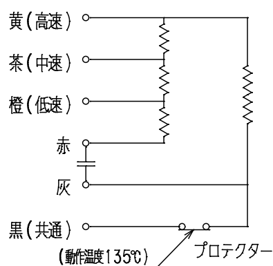
配線図
