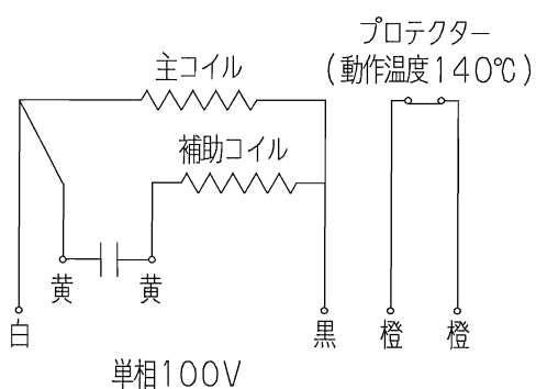
配線図
