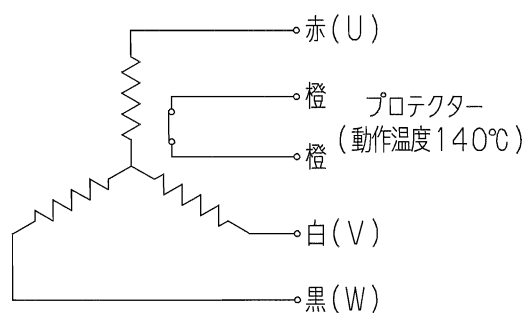
配線図
