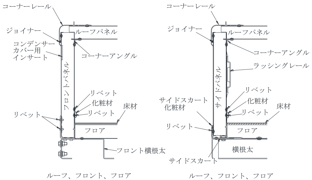
コンテナの構造概略図. 3
