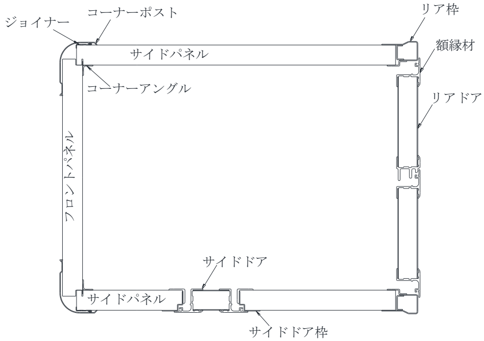
コンテナの構造概略図. 2
